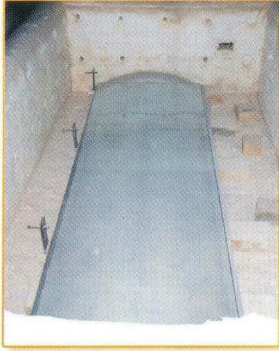
Verre plat posé sur un moule métallique dans le four avant bombage
