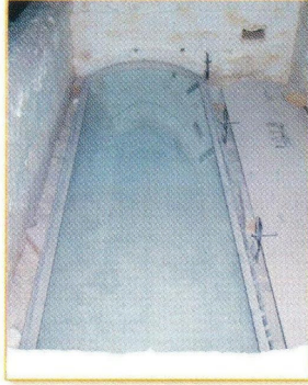
Verre plat posé sur un moule métallique dans le four après bombage
